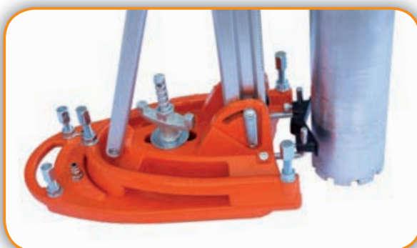
Bohrständer mit Vakuumplatte
