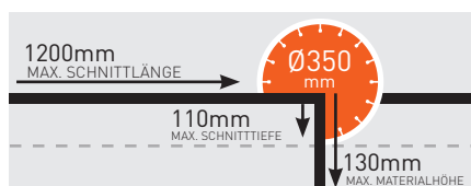
MAX. SCHNITTLÄNGE (mm) - CST 120
