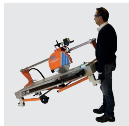
LEICHTER TRANSPORT DANK EINKLAPPBARER FÜSSE UND TRANSPORTRÄDER.
