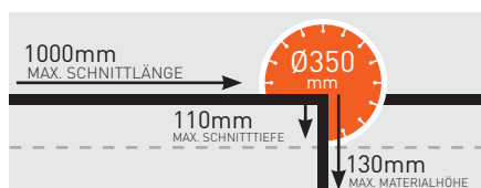
MAX. SCHNITTLÄNGE (mm) - CST 100
